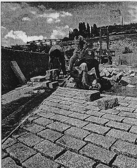
Obras en el Puente Mayor de Ciudad Rodrigo, incluidas en el periodo 2004-2006. VICENTE
