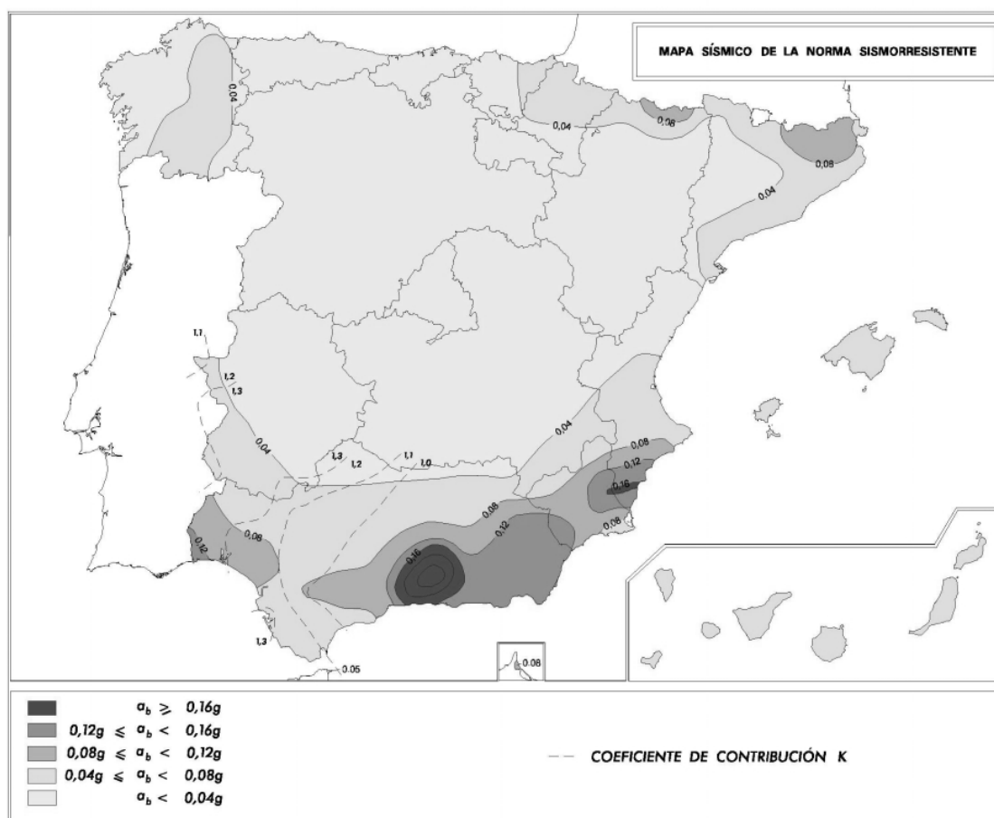
Figura 2.1. – Mapa de Peligrosidad Sísmica del el RD 997/2002
