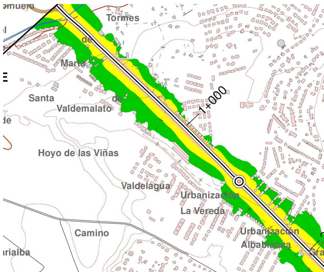
Niveles sonoros LNoche Sector UZ-7
